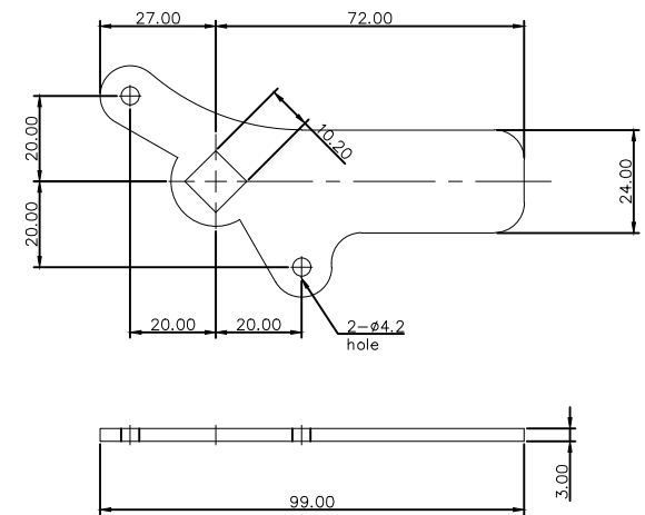
플레이트 (S-3)
