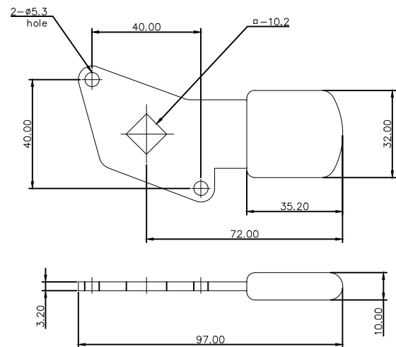
플레이트 (P-1-72)
