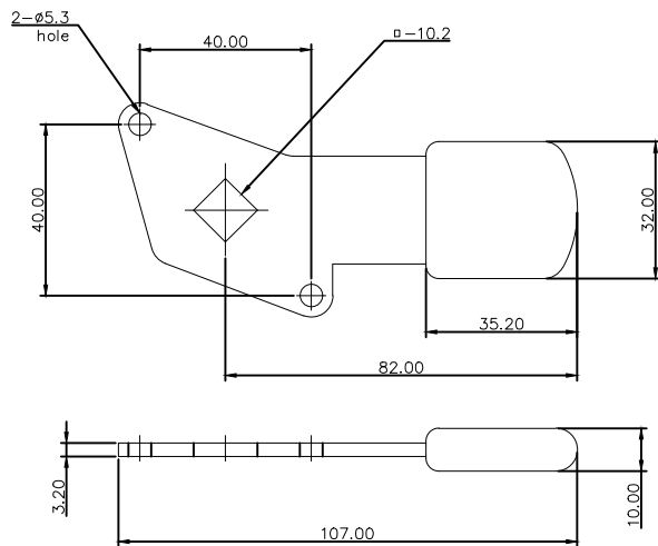
플레이트 (P-1-82)
