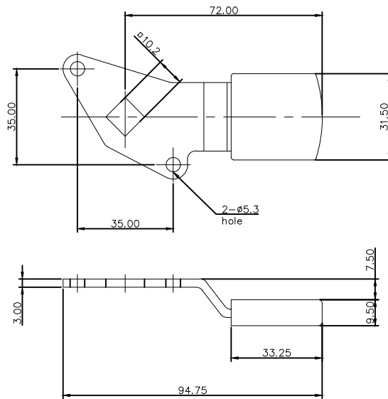
플레이트 (P-7)
