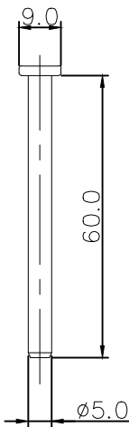
MS-5-60-L
