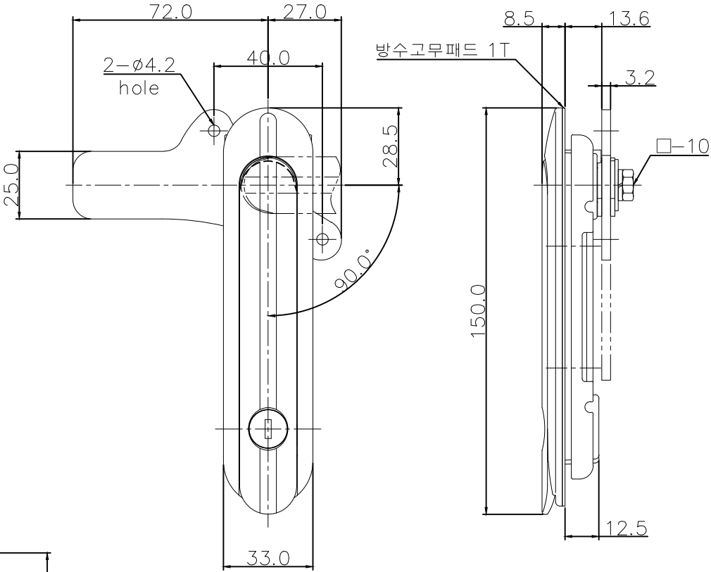
플레이트 (S-3) 조립예시
