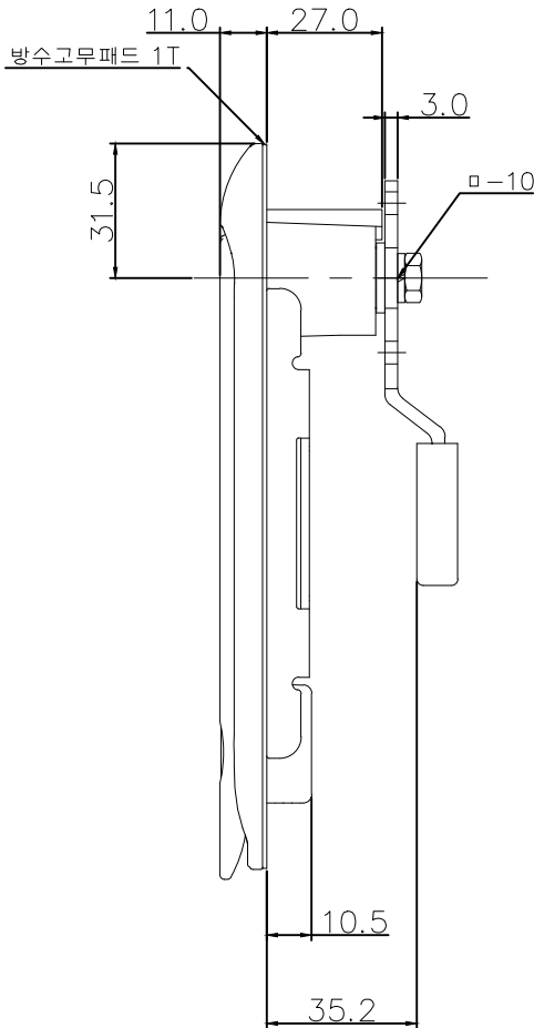
플레이트 (P-7) 조립예시
