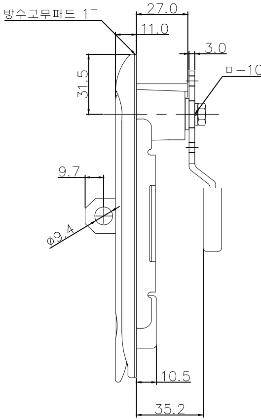
플레이트 (P-7) 조립예시
