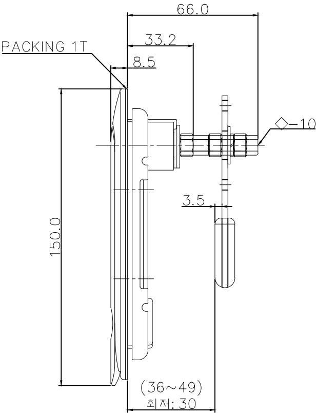
플레이트 (P-1-72) 조립예시
