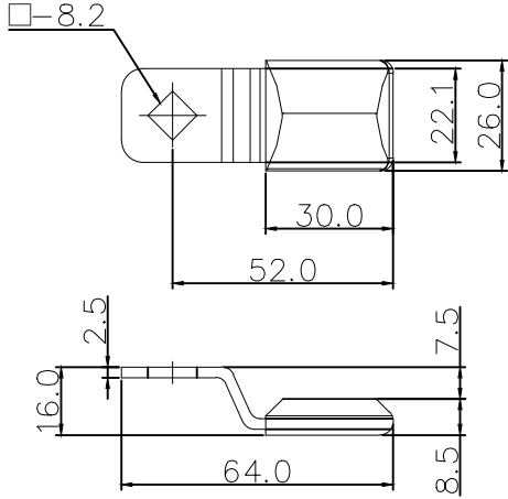
플레이트(P-5)
