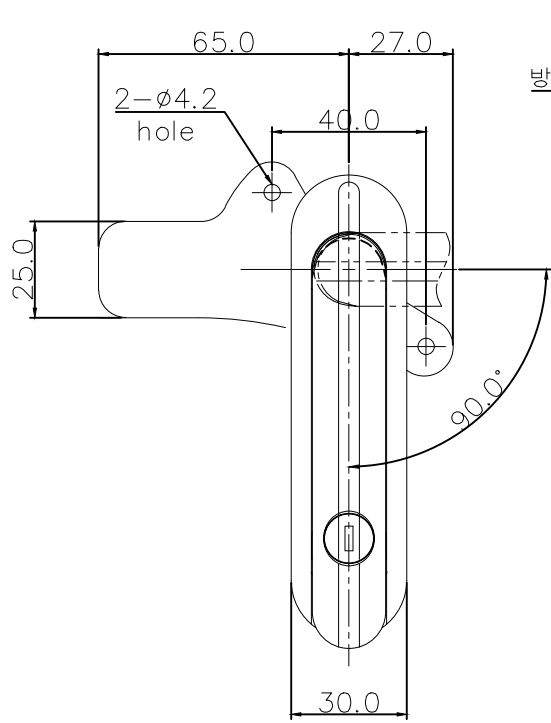
플레이트(P-5)
