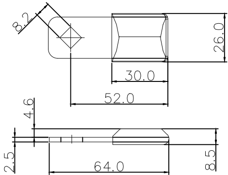
플레이트(P-3)
