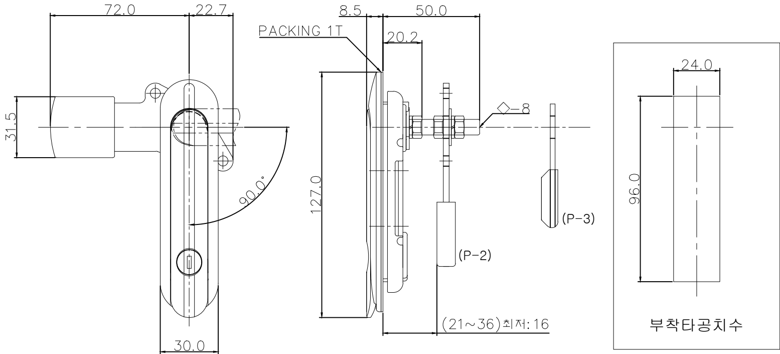
플레이트(P-2) 조립예시
