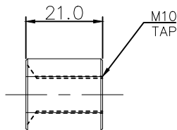
A-43-3T(M10)
