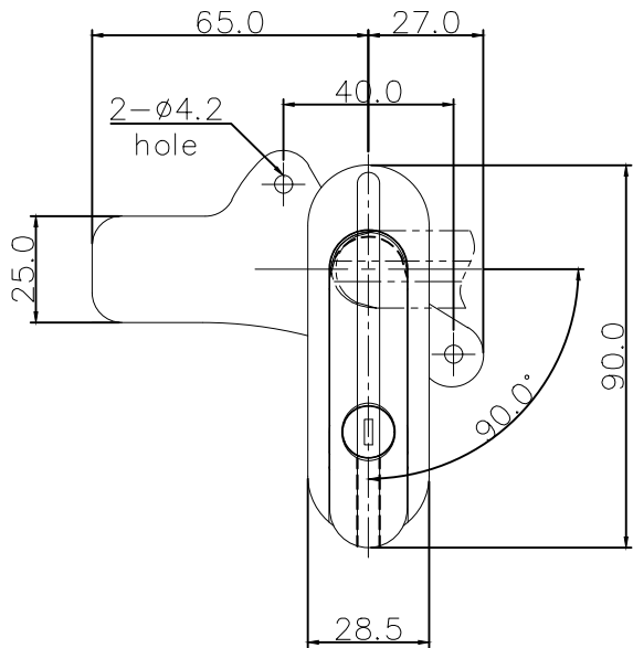
플레이트 (S-4) 조립예시
