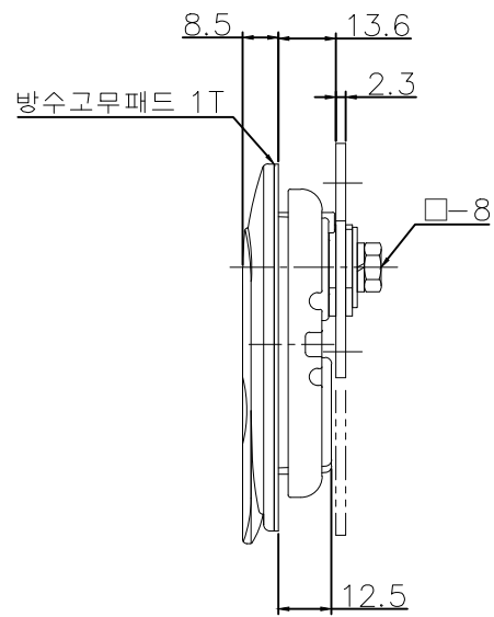
플레이트 (S-4) 조립예시
